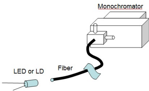
圖五 光頻量測實驗裝置圖
