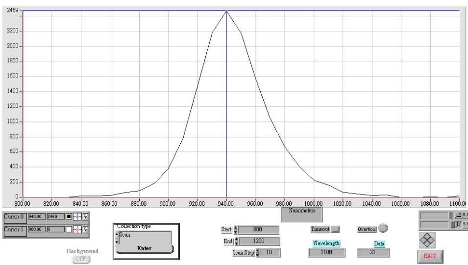
圖六(e) 點擊“Enter”，即開始偵測。偵測後光譜圖除了標示出中心波長之外，在圖的正上方也有半高寬(FWHM)的標示。
