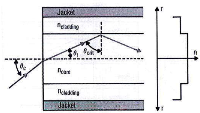
圖二 步階式光纖
