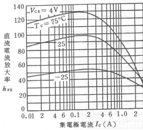
圖十四 2SC1060 的 h_{FE} 特性
