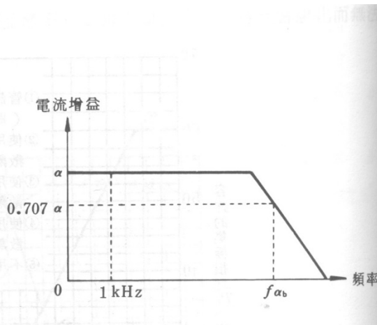
圖十五 高頻時電流增益會下降
